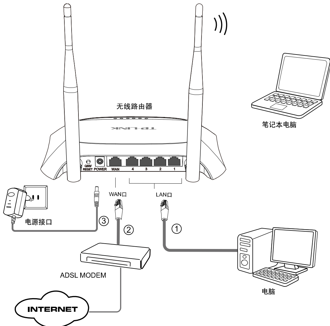
图 4-1 TL-WR845N 硬件安装示意图
