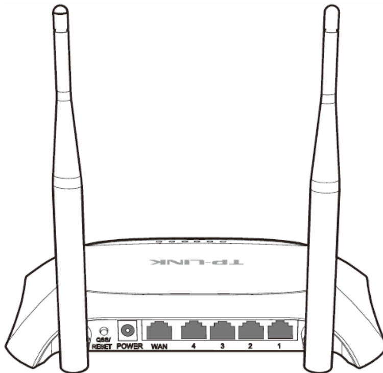
图 3-2 TL-WR845N 后面板示意图
